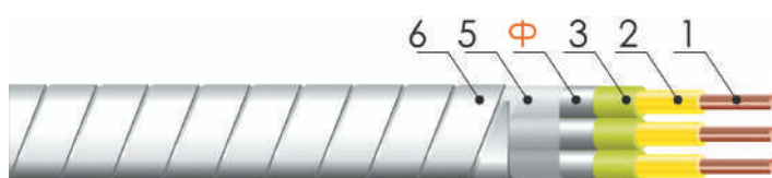
Усовершенствованная конструкция: кабель марки КПсПпФБП, КПсПФБП
