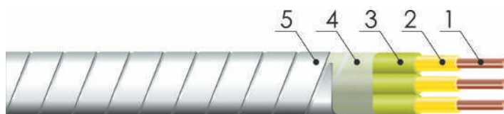
Базовая конструкция: кабель марки КПсПпБП, КПсПБП
