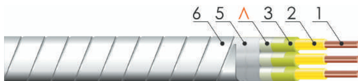
Усовершенствованная конструкция: кабель марки КПсПпЛБП, КПсПЛпБП
